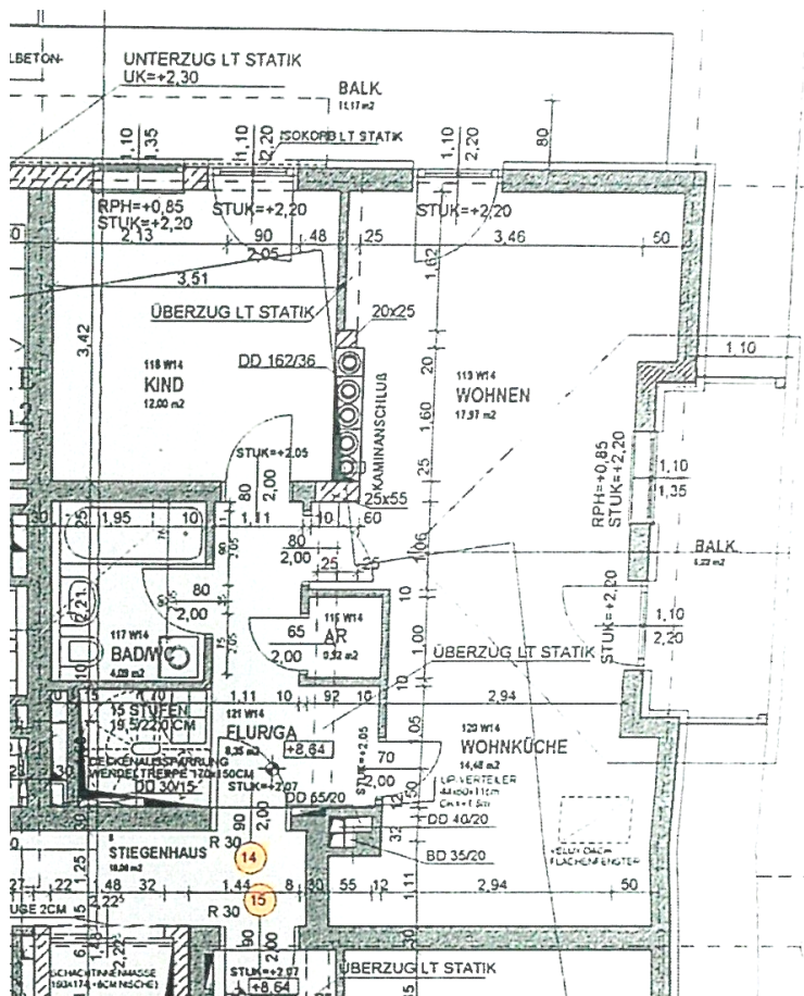
EINGANGSEBENE
