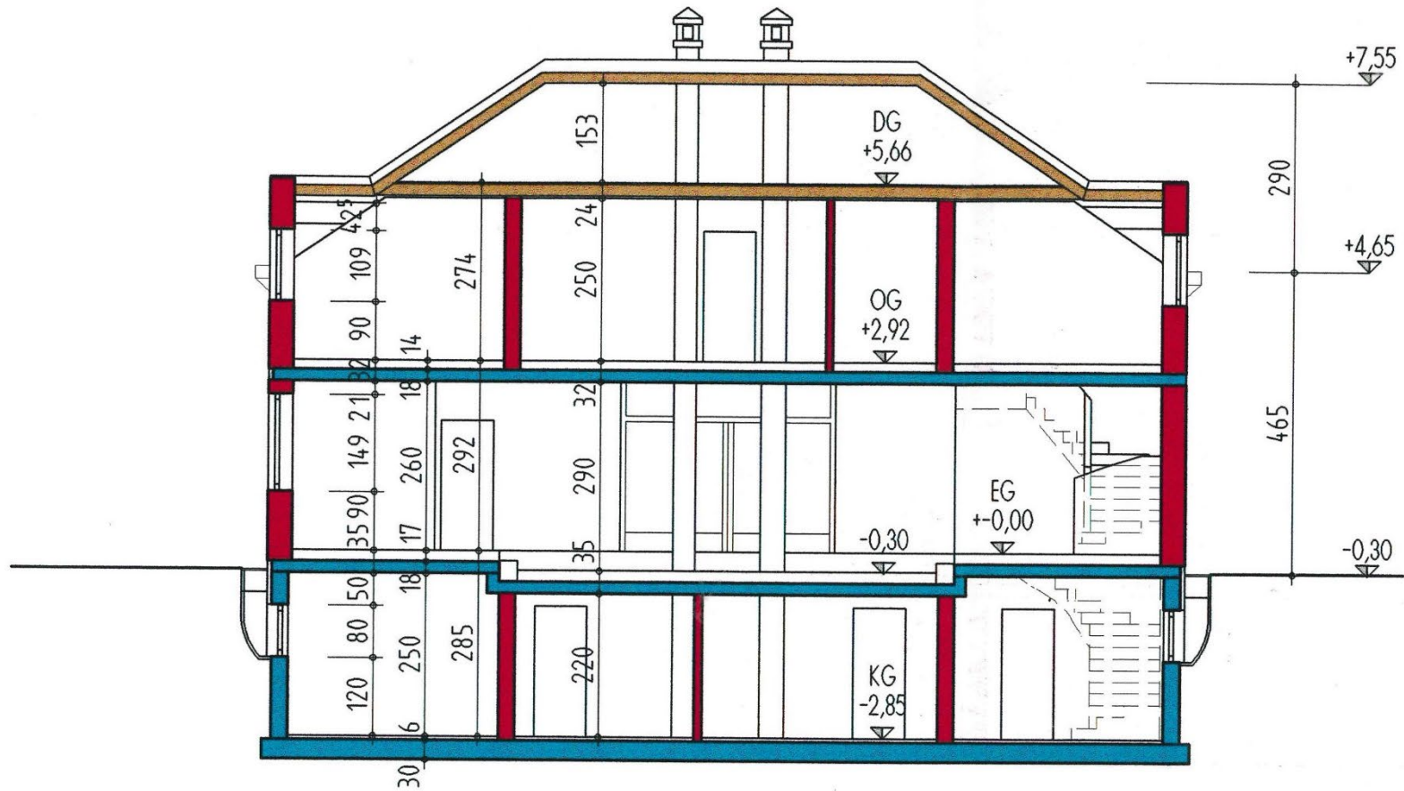
SCHNITT A-A
